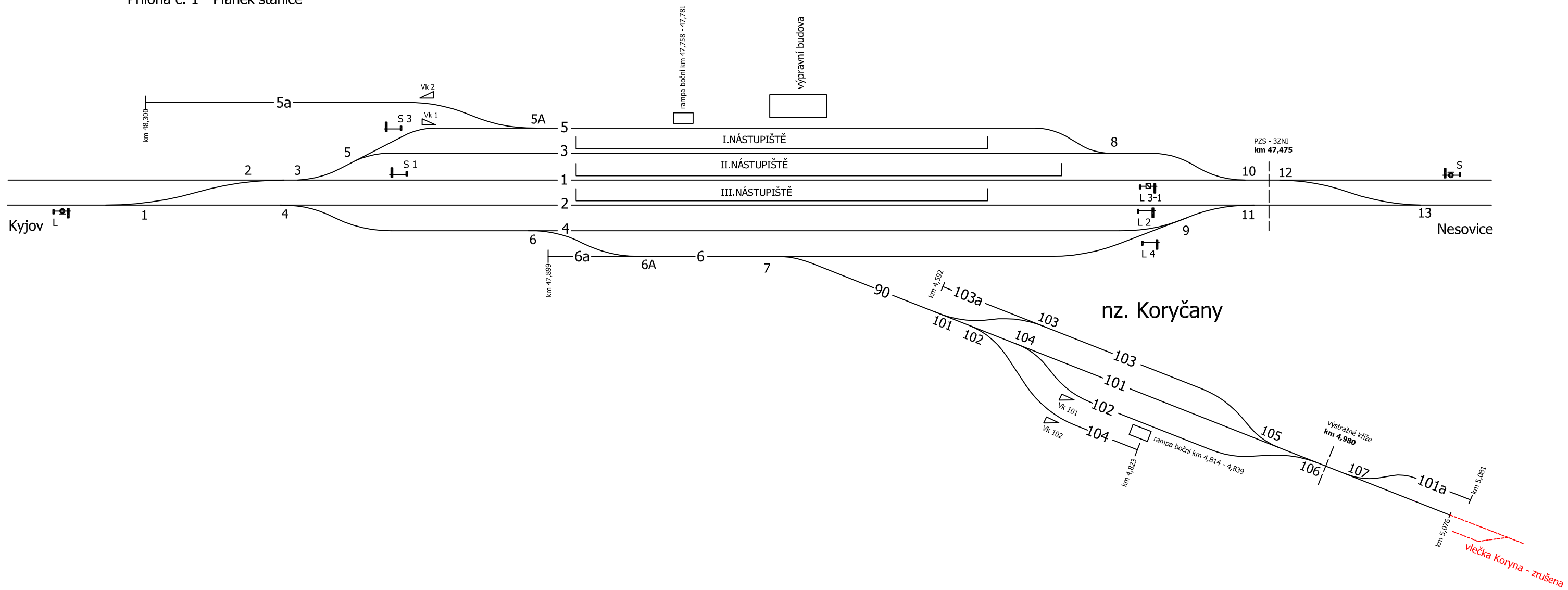
Příloha č. 1 - Plánek stanice
